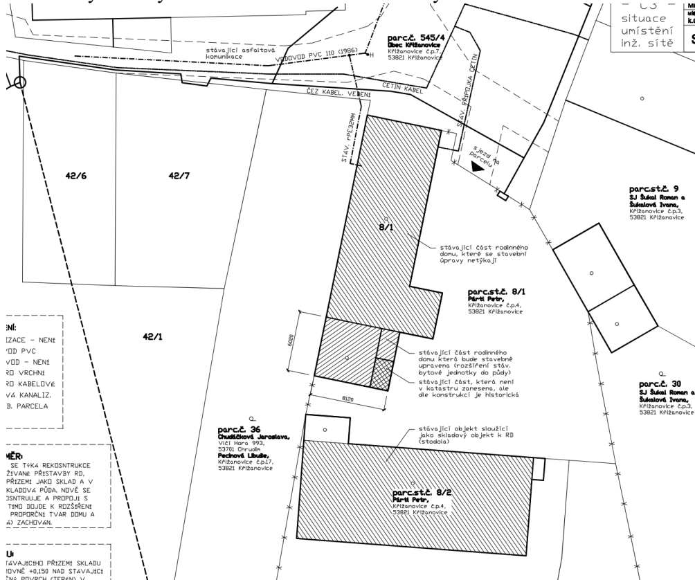
Situační výkres: Výřez z koordinačního situačního výkresu C.3
